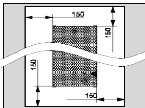
Рисунок 5.2 - Размеры размещения резистора в монтажном шкафу
