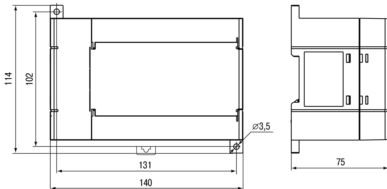
Рисунок 4.2 – Габаритные и установочные размеры прибора MB110-224.4ТД
