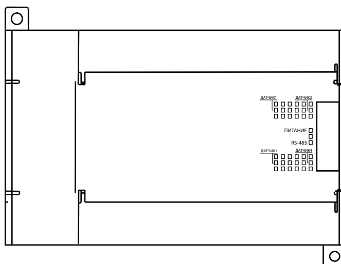
Рисунок 7.2 – Лицевая панель MB110-224.4ТД
