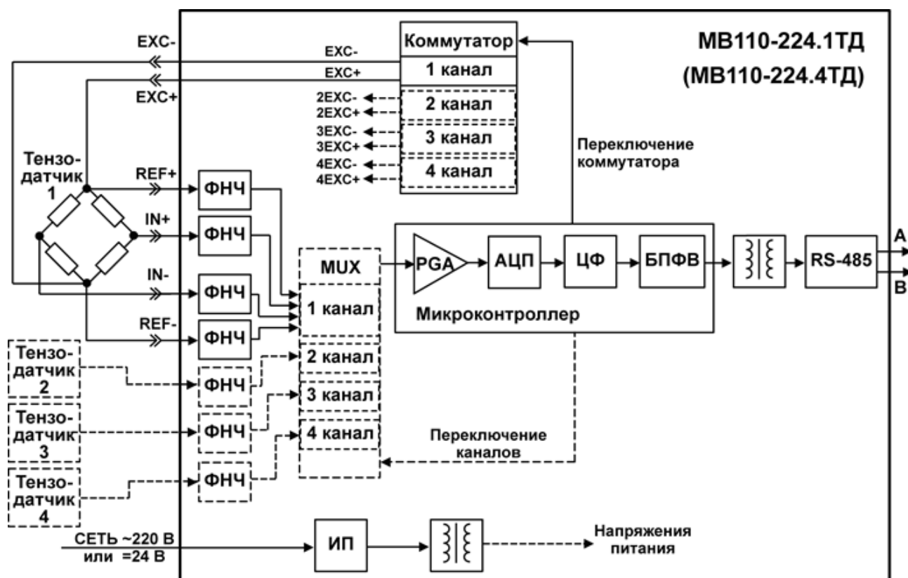
Рисунок 6.1 – Структурная схема прибора
