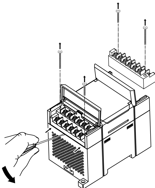
Рисунок 4.3 – Отделение клеммной колодки от прибора MB110-224.1ТД
