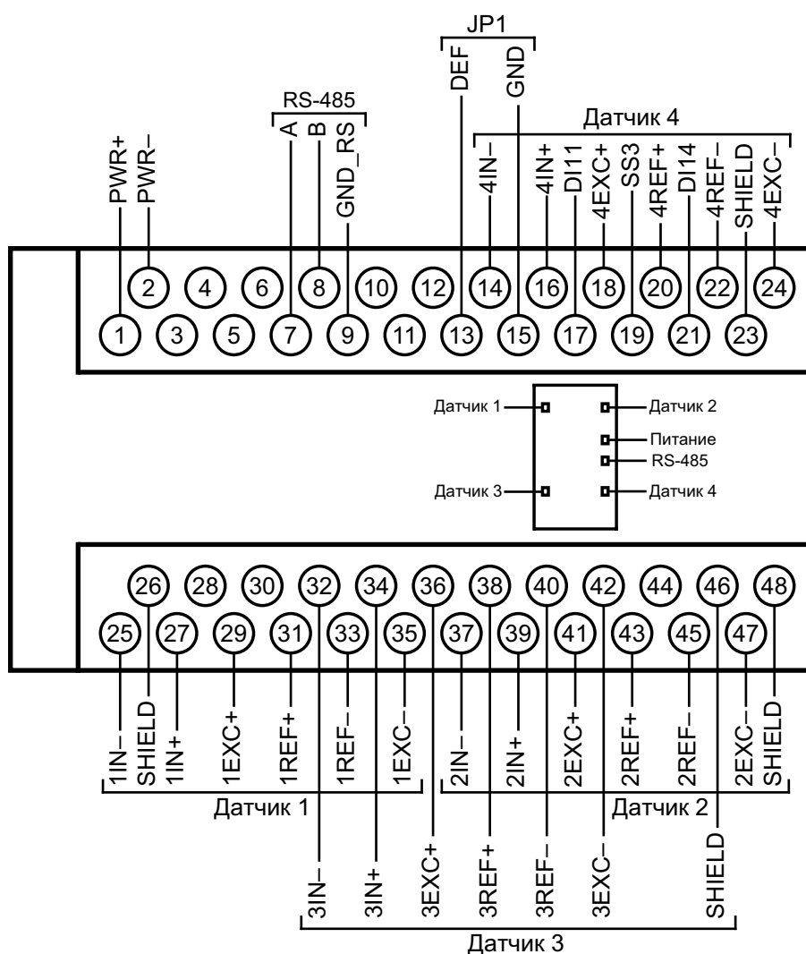
Рисунок 5.3 – Назначение контактов клеммной колодки MB110-224.4ТД
