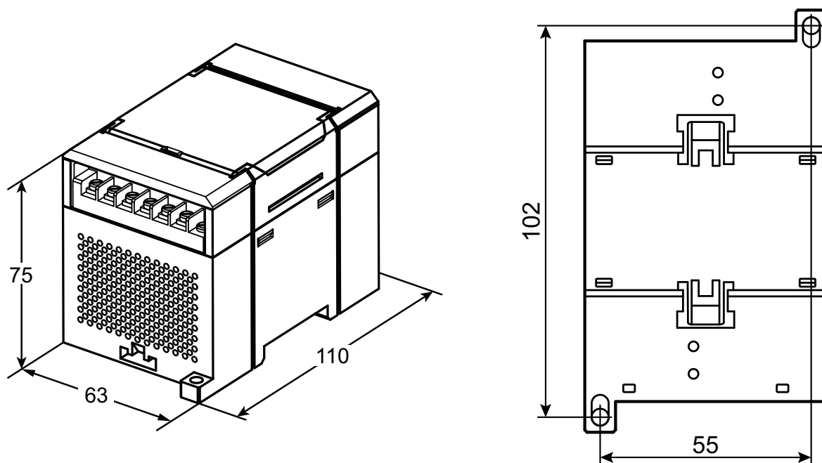
Рисунок 4.1 – Габаритные и установочные размеры прибора MB110-224.1ТД
