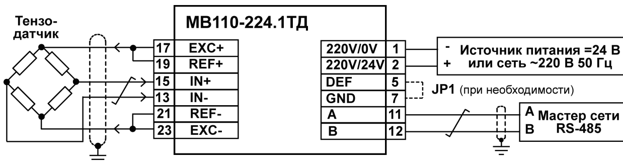
Рисунок 5.4 – Подключение к прибору MB110-224.1ТД внешних устройств с применением четырехпроводной схемы подключения к датчику и использованием заземления
