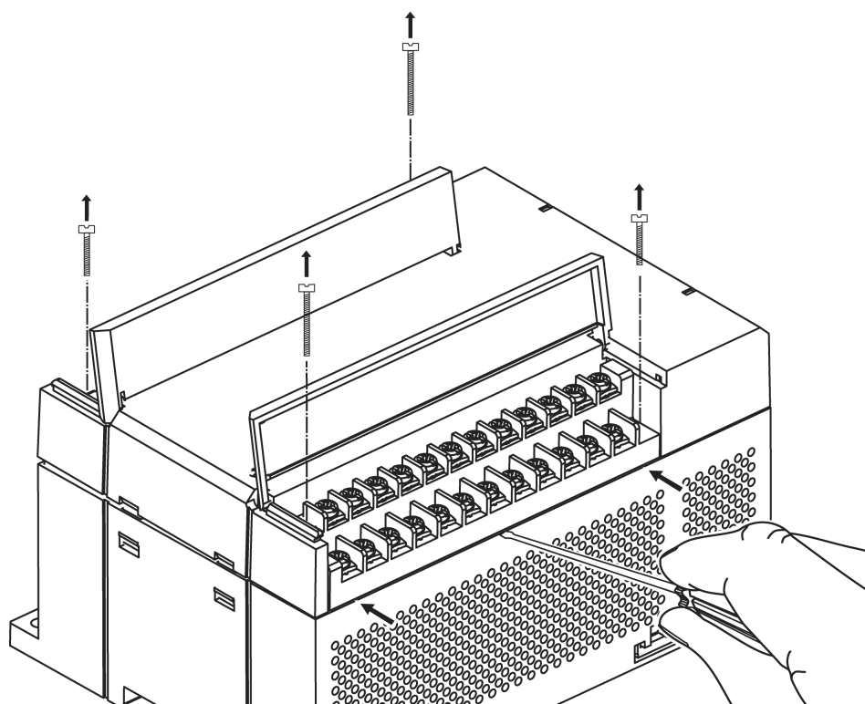
Рисунок 4.4 – Отделение клеммной колодки от прибора MB110-224.4ТД
