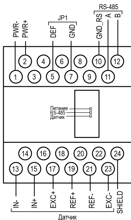
Рисунок 5.2 – Назначение контактов клеммной колодки MB110-224.1ТД
