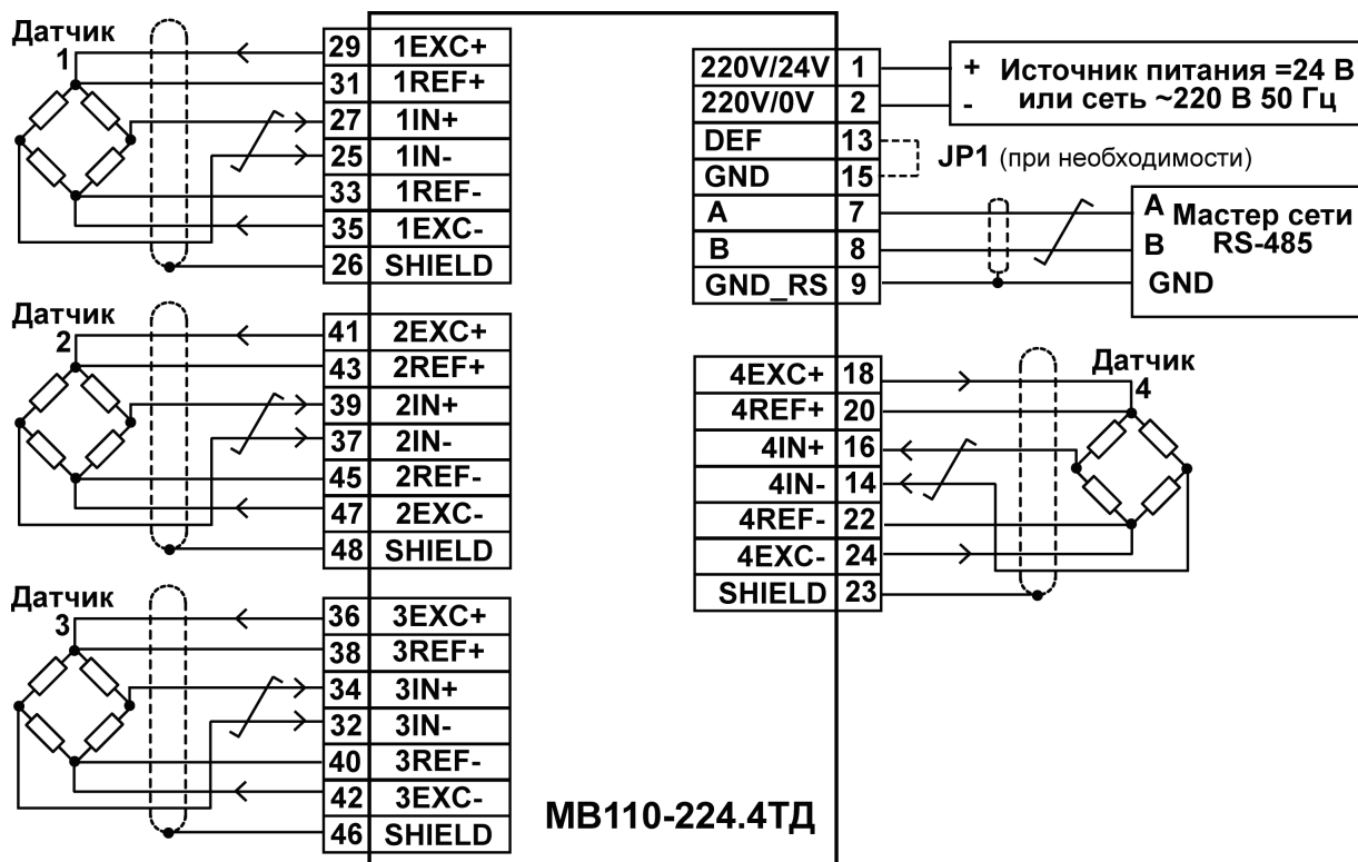
Рисунок 5.5 – Подключение к MB110-224.4ТД внешних устройств с применением шестипроводной схемы подключения к датчику и без использования заземления
