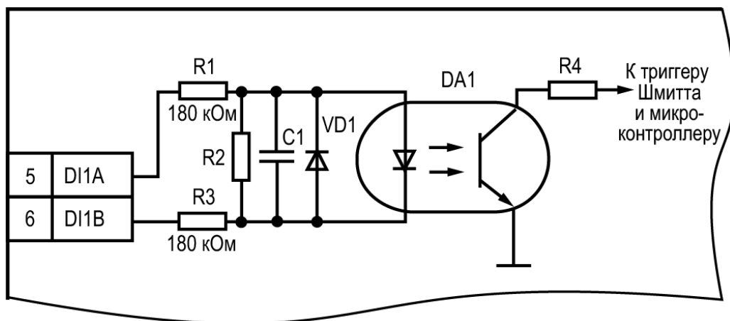
Рисунок 5.3 – Электрическая принципиальная схема входа (схемы других входов идентичны приведенной)
