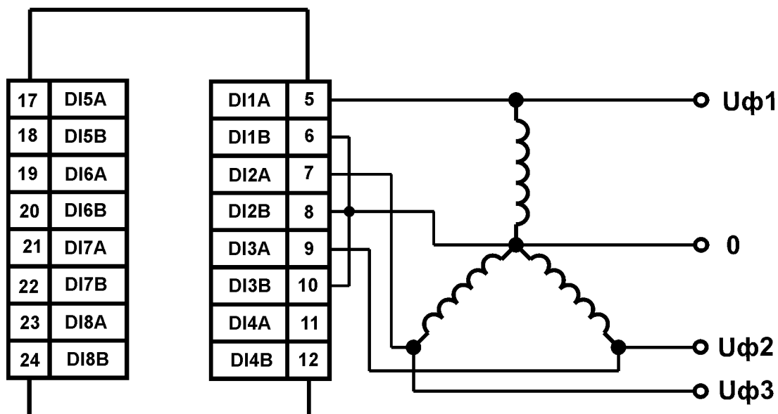
Рисунок 5.6 – Схема подключения трехфазного двигателя (пример контроля обрыва питающих фаз)
