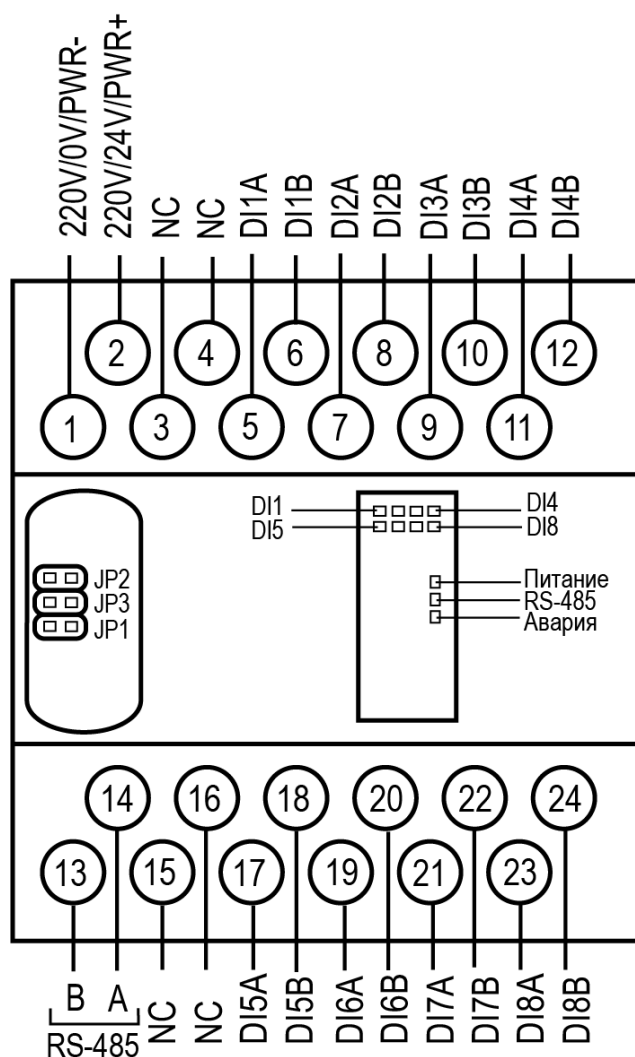
Рисунок 5.2 – Назначение контактов клеммника
