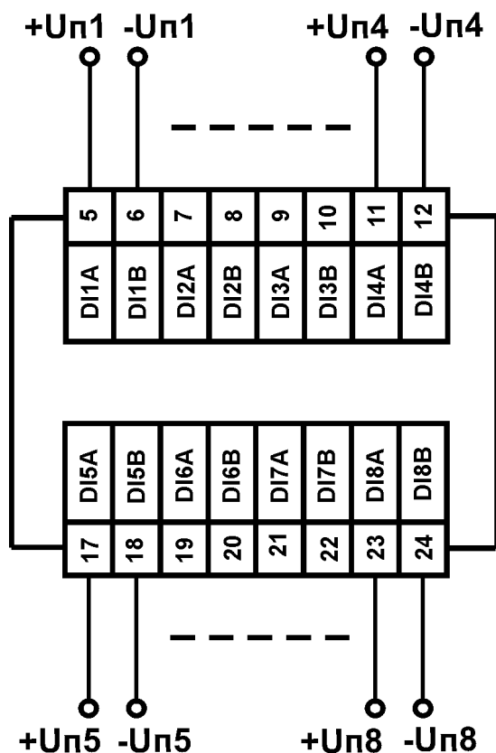
Рисунок 5.4 – Схема подключения сигналов постоянного напряжения
