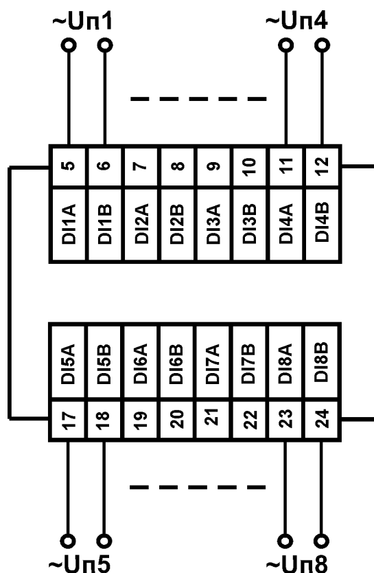
Рисунок 5.5 – Схема подключения сигналов переменного напряжения
