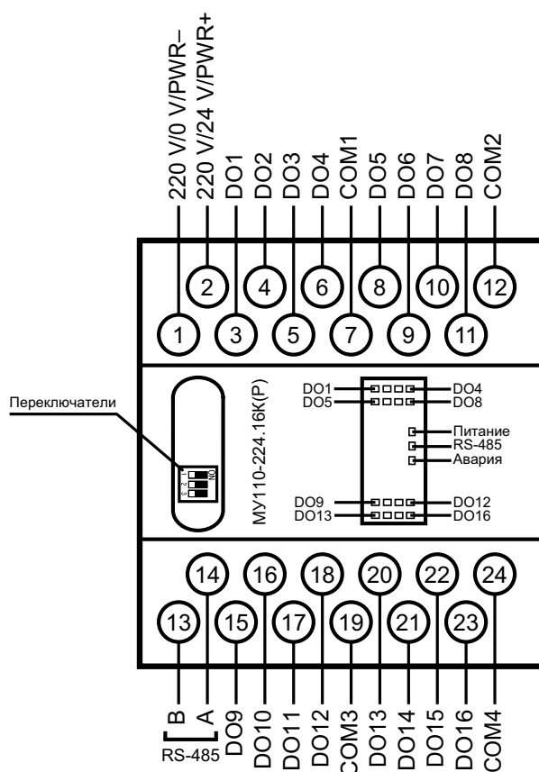
Рисунок 5.2 – Назначение контактов клеммника MY110-224.16K и MY110-224.16P
