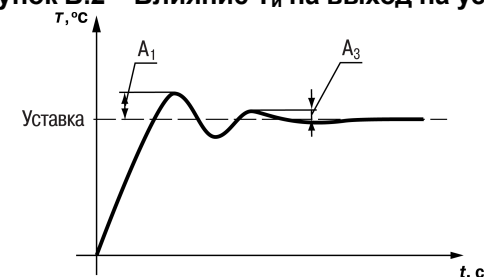
Рисунок Б.3 – Оценка ошибки регулирования
