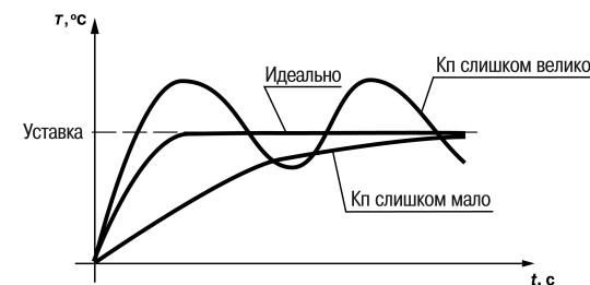
Рисунок Б.1 – Влияние K_{\Pi} на выход на уставку
