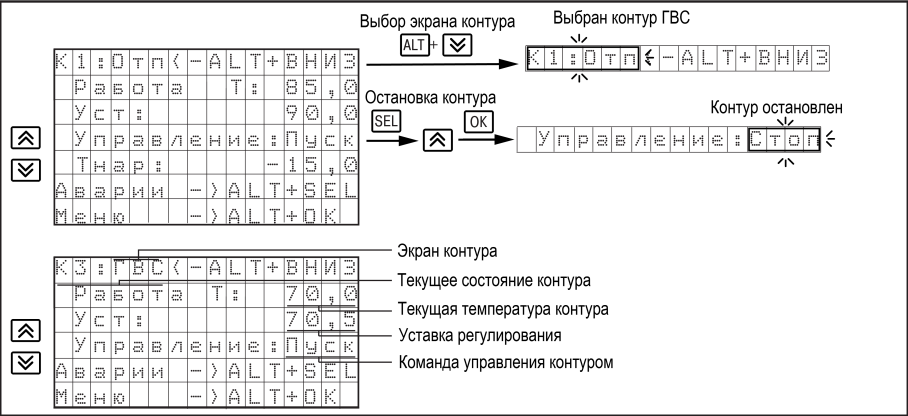
Рисунок 7.2 – Главный экран
