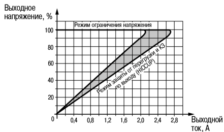
Рисунок 3 – График зависимости выходного напряжения от выходного тока (НСССР)
