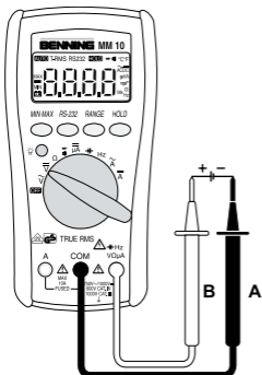
Bild 2: Gleichspannungsmessung Fig. 2: Direct voltage measurement Fig. 2: Mesure de tension continue Fig. 2: Medición de tensión continua obr. 2: Měření stejnosměrného napětí figura 2: DC-μέτρηση ill. 2: Misura tensione continua Fig. 2: Meten van gelijkspanning Rys. 2: Pomiar napięcia stałego Imaginea 2: Măsurarea tensiunii continue рис. 2: Измерение напряжения постоянного тока Fig. 2: Likspänningsmätning Resim 2: Doğru Gerilim Ölçümü
