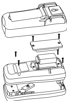
Bild 12: Sicherungswechsel Fig. 12: Fuse replacement Fig. 12: Remplacement des fusibles Fig. 12: Cambio de fusible obr. 12: Výměna pojistek фигура 12: αντικατάσταση ασφάλειας ill. 12: Sostituzione fusibile Fig. 12: Vervanging van de smeltzekeringen Rys. 12: Wymiana bezpiecznika Imaginea 12: Schimbarea siguranțelor рис. 12: Замена предохранителей Fig. 12: Säkkringsbyte Resim 12: Sigorta Değişimi
