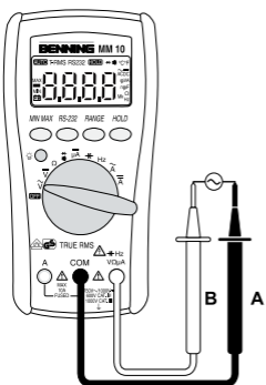
Bild 3: Wechselspannungsmessung Fig. 3: Alternating voltage measurement Fig. 3: Mesure de tension alternative Fig. 3: Medición de tensión alterna obr. 3: Měření střídavého napětí figura 3: AC μέτρηση ill. 3: Misura tensione alternata Fig. 3: Meten van wisselspanning Rys. 3: Pomiar napięcia przemiennego Imaginea 3: Măsurarea tensiunii alternative рис. 3: Измерение напряжения переменного тока Fig. 3: Växelspänningsmätning Resim 3: Alternatif Gerilim Ölçümü
