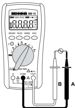
Bild 10: Frequenzmessung Fig. 10: Frequency measurement Fig. 10: Mesure de fréquence Fig. 10: Medición de frecuencia obr. 10: Měření frekvence фигура 10: Μέτρηση συχνότητας ill. 10: Misura di frequenza Fig. 10: Frequentiemeting Rys.10: Pomiar częstotliwości Imaginea 10: Măsurarea frecvenței рис. 10: Измерение частоты Fig. 10: Frekvensmätning Resim 10: Frekans Ölçümü
