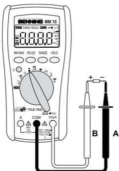
Bild 8: Durchgangsprüfung mit Summer Fig. 8: Continuity Testing with buzzer Fig. 8: Contrôle de continuité avec ronfleur Fig. 8: Control de continuitad con vibrador obr. 8: Zkouška obvodu фигура 8: Έλεγχος συνέχειας με βομβητή ill. 8: Prova di continuità con cicalino Fig. 8: Doorgangstest met akoestisch signaal Rys.8: Sprawdzenie ciągłości obwodu Imaginea 8: Verificarea continuității cu buzzer рис. 8: Проверка целостности цепи Fig. 8: Genomgångstest med summer Resim 8: Sesli ulyarici ile süreklilik ölçümü
