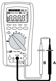
Bild 6: Widerstandsmessung Fig. 6: Resistance measurement Fig. 6: Mesure de résistance Fig. 6: Medición de resistencia obr. 6: Měření odporu figura 6: Μέτρηση αντίστασης ill. 6: Misura di resistenza Fig. 6: Weerstandsmeting Rys.6: Pomiar rezystancji Imaginea 6: Măsurarea rezistenței рис. 6: Измерение сопротивления Fig. 6: Resistansmätning Resim 6: Direnç Ölçümü
