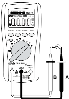
Bild 5: Wechselstrommessung Fig. 5: AC current measurement Fig. 5: Mesure de courant alternatif Fig. 5: Medición de corriente alterna obr. 5: Měření střídavého proudu figura 5: AC-μέτρηση ill. 5: Misura corrente alternata Fig. 5: Meten van wisselstroom Rys.5: Pomiar prądu przemiennego Imaginea 5: Măsurarea curentului alternativ рис. 5: Измерение величины переменного тока Fig. 5: Växelströmsmätning Resim 5: Alternatif Akım Ölçümü
