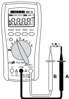
Bild 7: Diodenprüfung Fig. 7: Diode Testing Fig. 7: Contrôle de diodes Fig. 7: Verificación de diodos obr. 7: test diod figura 7: Έλεγχος διόδου ill. 7: Prova diodi Fig. 7: Diod-test Rys.7: Pomiar diody Imaginea 7: Testarea diodelor рис. 7: Проверка диодов Fig. 7: Diodecontrole Resim 7: Diyot Kontrolü
