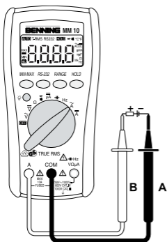
Bild 4: Gleichstrommessung Fig. 4: DC current measurement Fig. 4: Mesure de courant continu Fig. 4: Medición de corriente continua obr. 4: Měření stejnosměrného proudu figura 4: DC-μέτρηση ill. 4: Misura corrente continua Fig. 4: Meten van gelijkstroom Rys. 4: Pomiar prądu stałego Imaginea 4: Măsurarea curentului continuu рис. 4: Измерение величины постоянного тока Fig. 4: Likströmsmätning Resim 4: Doğru Akım Ölçümü
