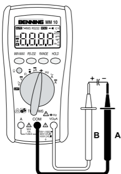
Bild 9: Kapazitätsmessung Fig. 9: Capacity Testing Fig. 9: Mesure de capacité Fig. 9: Medición de capacidad obr. 9: Měření kapacity фигура 9: Μέτρηση χωρητικότητας ill. 9: Misura di capacità Fig. 9: Capaciteitsmeting Rys.9: Pomiar pojemności Imaginea 9: Măsurarea capacității рис. 9: Измерение емкости Fig. 9: Karacitansmätning Resim 9: Kapasite Ölçümü
