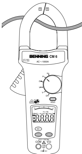
Bild 4: Wechselstrommessung Fig. 4: AC current measurement Fig. 4: Mesure de courant alternatif Fig. 4: Medición de corriente alterna obr. 4: Měření střídavého proudu σχήμα 4: Μέτρηση εναλλασσόμενης έντασης ill. 4: Misura corrente alternata Fig. 4: Meten van wisselstroom Rys.4: Pomiar prądu przemiennego Imaginea 4: Măsurarea curentului alternativ рис. 4: Измерение величины переменного тока Fig. 4: Växelströmsmätning Resim 4: Alternatif Akım Ölçümü
