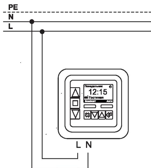
Рисунок 2. Схема подключения
