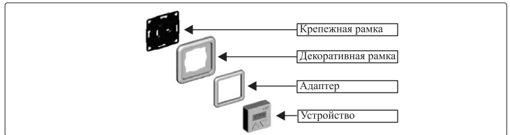
Рисунок 3. Крепление устройства
